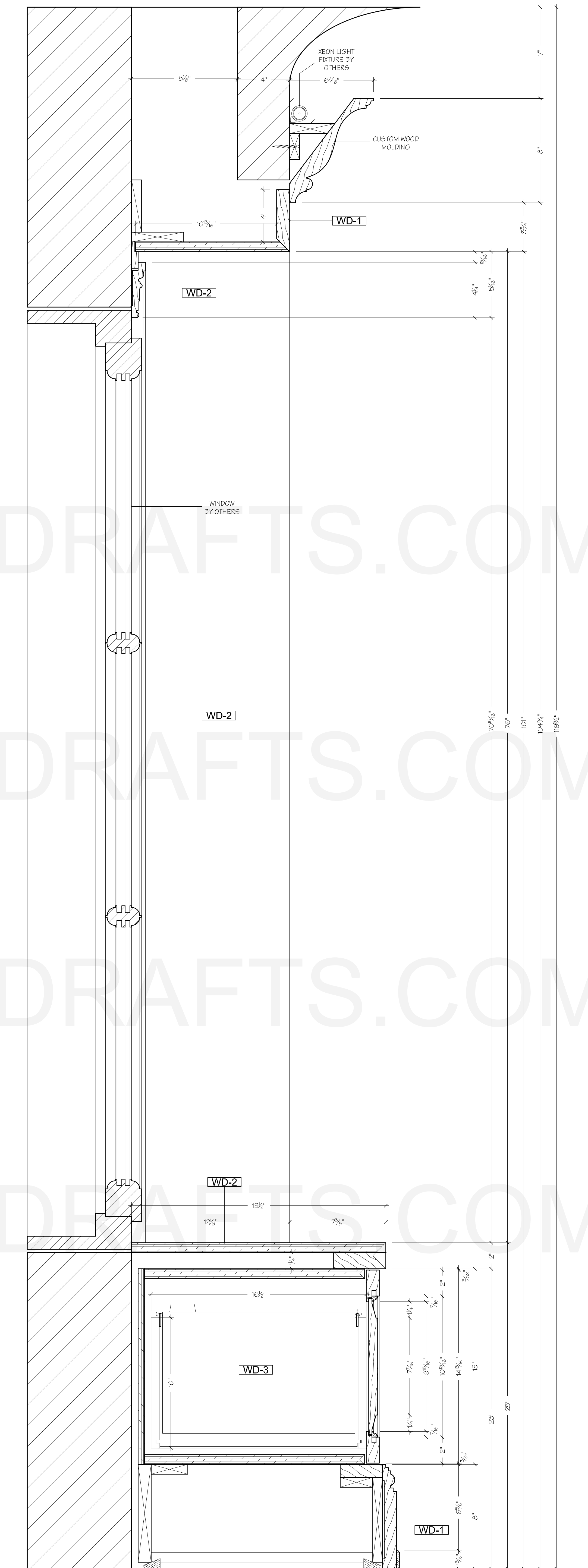
14 SECTION SCALE: 3" = 1'-0"
